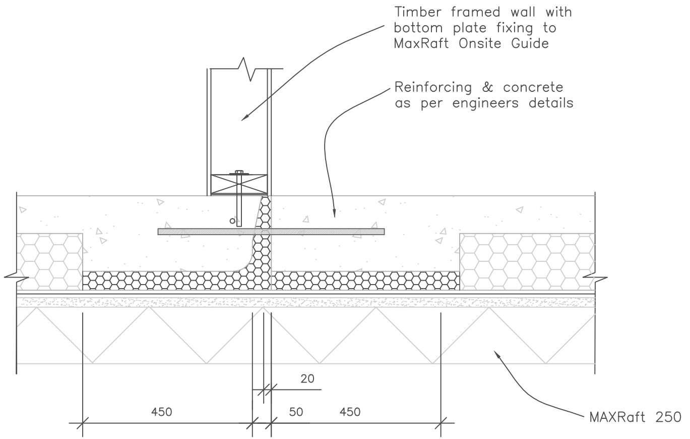
MAXRaft© 250 - Thermal break
